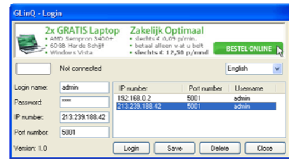
Afbeelding 1, Login scherm
